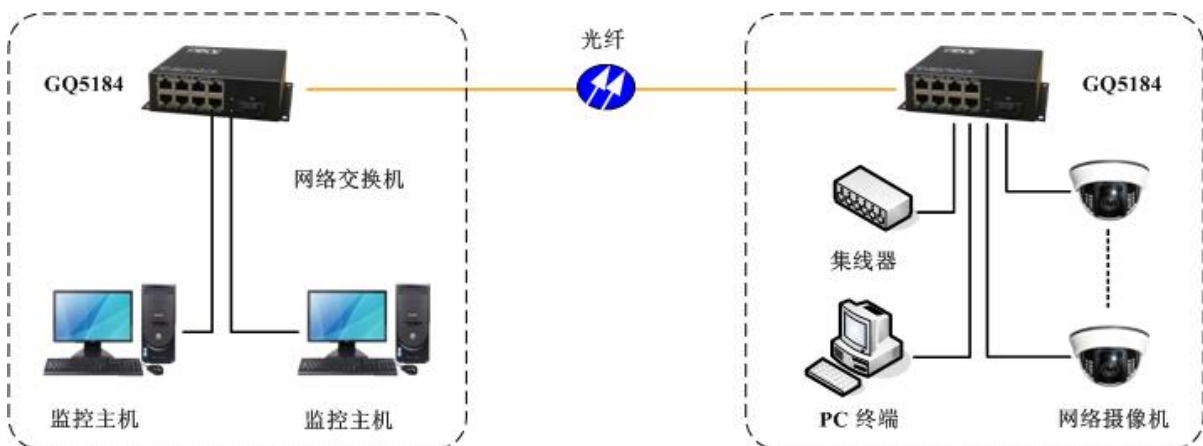
光纤点对点组网
