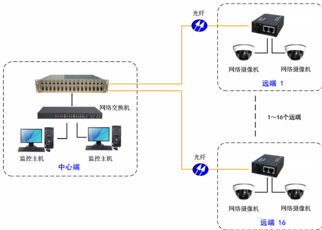
方案二：光纤点对多点组网
