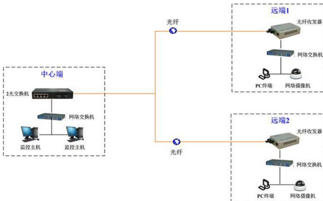
方案二：光纤1点对2点组网
